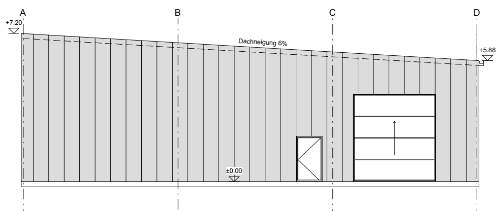
Seitenansicht Achse 1
