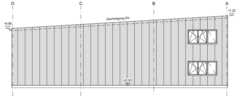
Seitenansicht Achse 8
